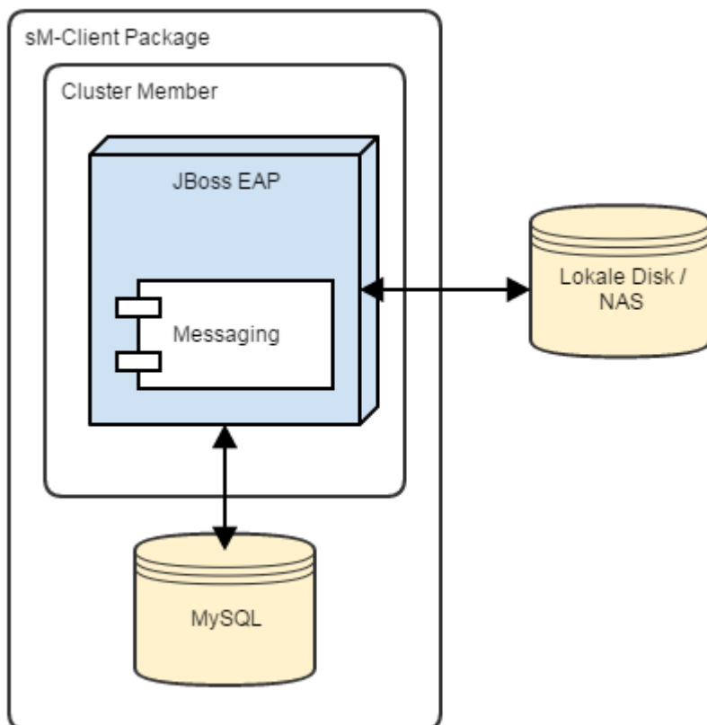
Abbildung 1 Referenzarchitektur
